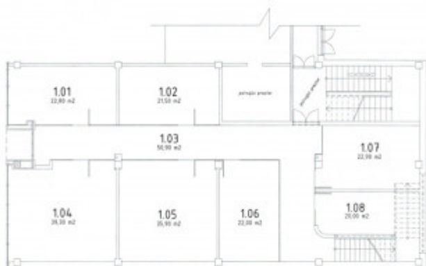
DOM OBCHODU A SLUŽIEB AFK - Pôdorys 1.N
